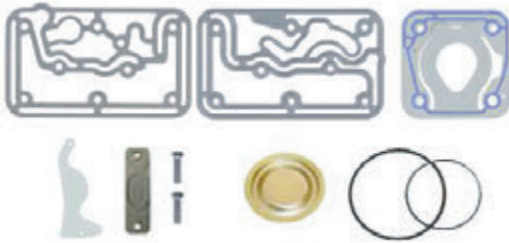
Kompresör Conta Takımı Compressor Gasket Kit 412 352 003 2
