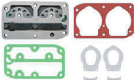
Kompresör Pleyt Tamir Compressor Plate Kit
