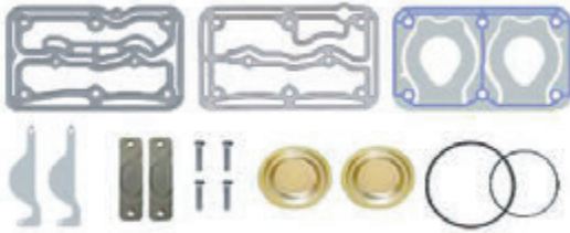
Kompresör Conta Takımı Compressor Gasket Kit 412 724 928 2
