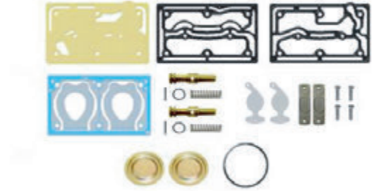
Kompresör Tamir Takımı Compressor Repair Kit
