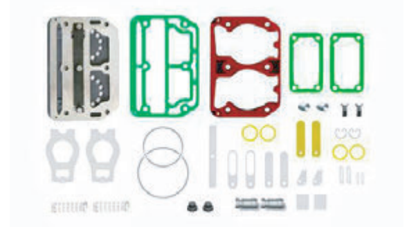
Kompresör Tamir Takımı Compressor Repair Kit
