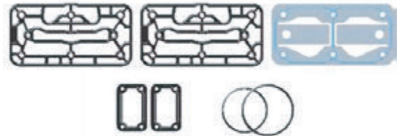
Kompresör Conta Takımı Compressor Gasket Kit 911 504 910 3
