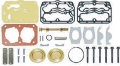
Kompresör Tamir Takımı Compressor Repair Kit 1737654
