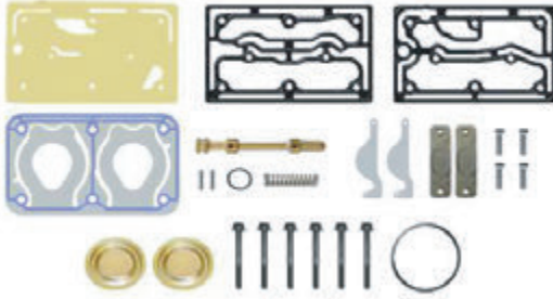
Kompresör Tamir Takımı Compressor Repair Kit
