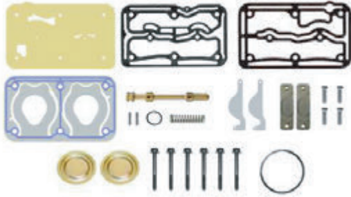
Kompresör Tamir Takımı Compressor Repair Kit 412 704 920 2
