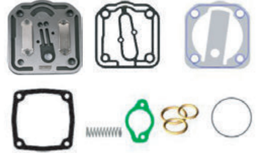
Kompresör Tamir Takımı Compressor Repair Kit 541 130 0820
