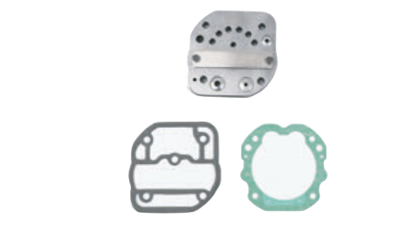
Kompresör Pleyt Tamir Compressor Plate Repair 411 033 505 2
