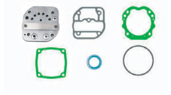
Kompresör Tamir Takımı Compressor Repair Kit 442 130 0120 - 81 54124 6013
