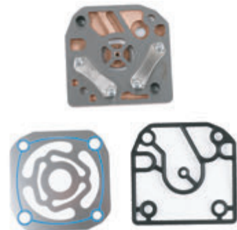
Kompresör Pleyt Tamir Compressor Plate Kit
