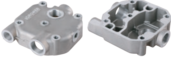
Üst Kapak Cylinder Head 442 130 3219
