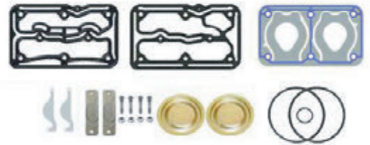
Kompresör Tamir Takımı Compressor Repair Kit 001 130 2315 - 001 130 2815
