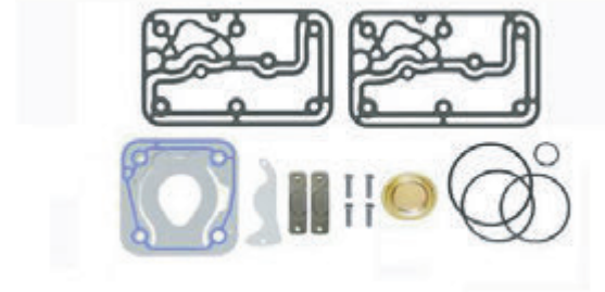
Kompresör Conta Takımı Compressor Gasket Kit
