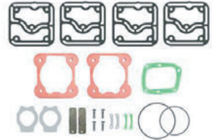
Kompresör Conta Takımı Compressor Gasket Kit 81541916954
