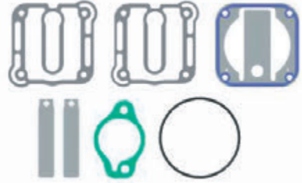
Kompresör Conta Takımı Compressor Gasket Kit
